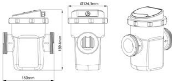
TKB 102, TKB 103 MÉRET
