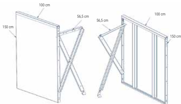
A PANALEK MÉRETEI
